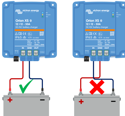
Beispiel für richtige und falsche (vertauschte) Batteriepolartät:
